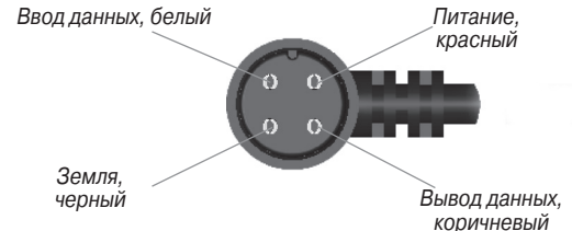
Вид кабеля
